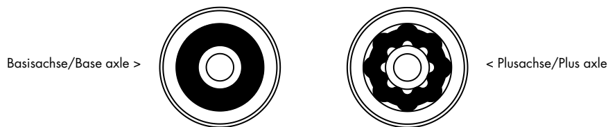
Fangtopf (sicht von oben) / Plan view of top insulator
